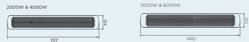
DECKENEINBAURAHMEN 2000W & 4000W
